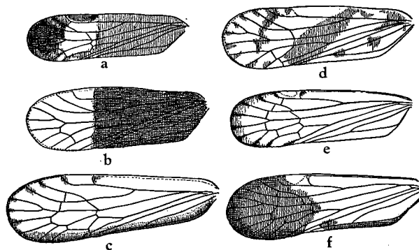
FIGURE 2.—a, Myndus bifurcatus , tegmen; b, M. dibaphus , tegmen; c, M. marginatus , tegmen; d, M. nearchus , tegmen; e, M. polycator , tegmen; f, M. niger , tegmen.
