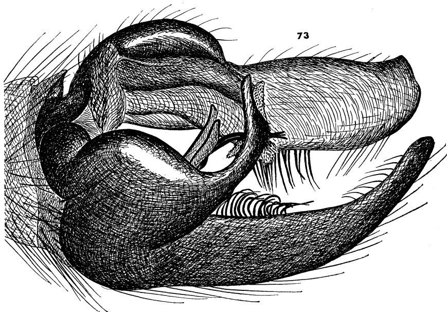
Fig. 73. Heligmonera spuria (Wulp), ♂ genitalia.
