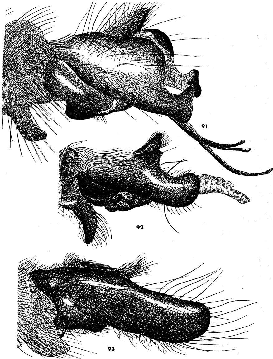
Fig. 91-93. Promachus , ♂ genitalia: 91, manilliensis (Macquart); 92, maculosus n. sp.; 93, leucopareus n. sp.
