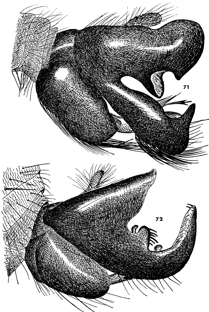
Fig. 71, 72. Heligmonera , ♂ genitalia: 71, divaricata n. sp.; 72, pygmaea n. sp.
