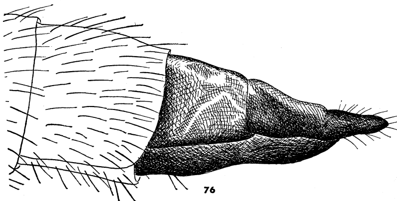
Fig. 74-76. Ovipositors. 74, Astochia scalaris Hermann; 75, Machimus aurentulus Becker; 76, Machimus divinosus n. sp.
