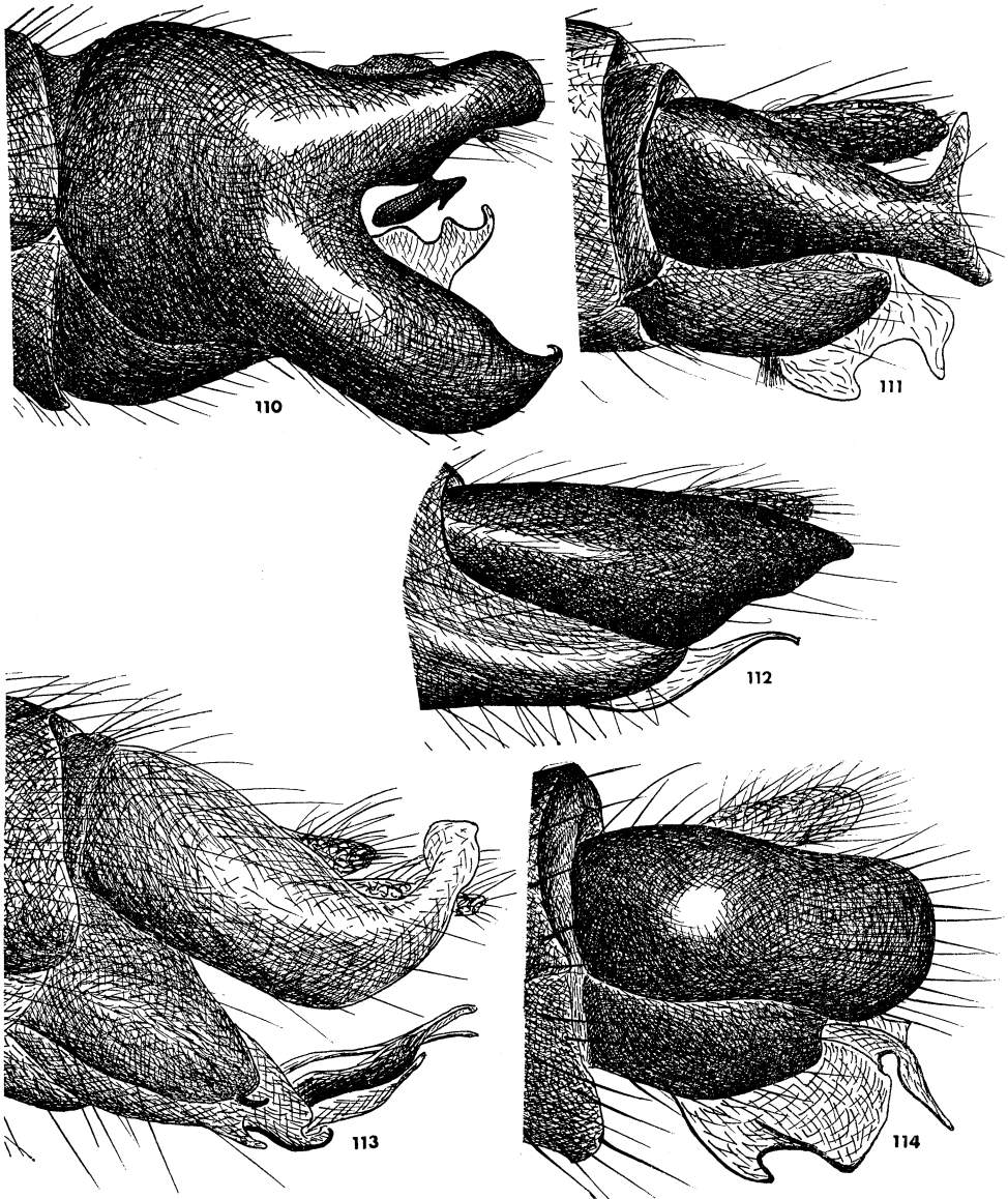
Fig. 110-114. Ommatius , ♂ genitalia. 110, episkeris n. sp. ; 111, docimus n. sp. ; 112, coptus n. sp. ; 113, manipulus n. sp. ; 114, suntius n. sp.
