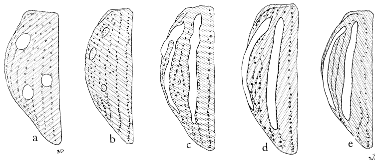
Fig. 15. Pantorhytes elytral diagrams: a, sexpustulatus Hllr, Finisterre Mts; b, pallidus n. sp.; c, irregularis n. sp.; d, manni n. sp.; e, arcuatus n. sp.
